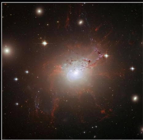
PERSEUS A
